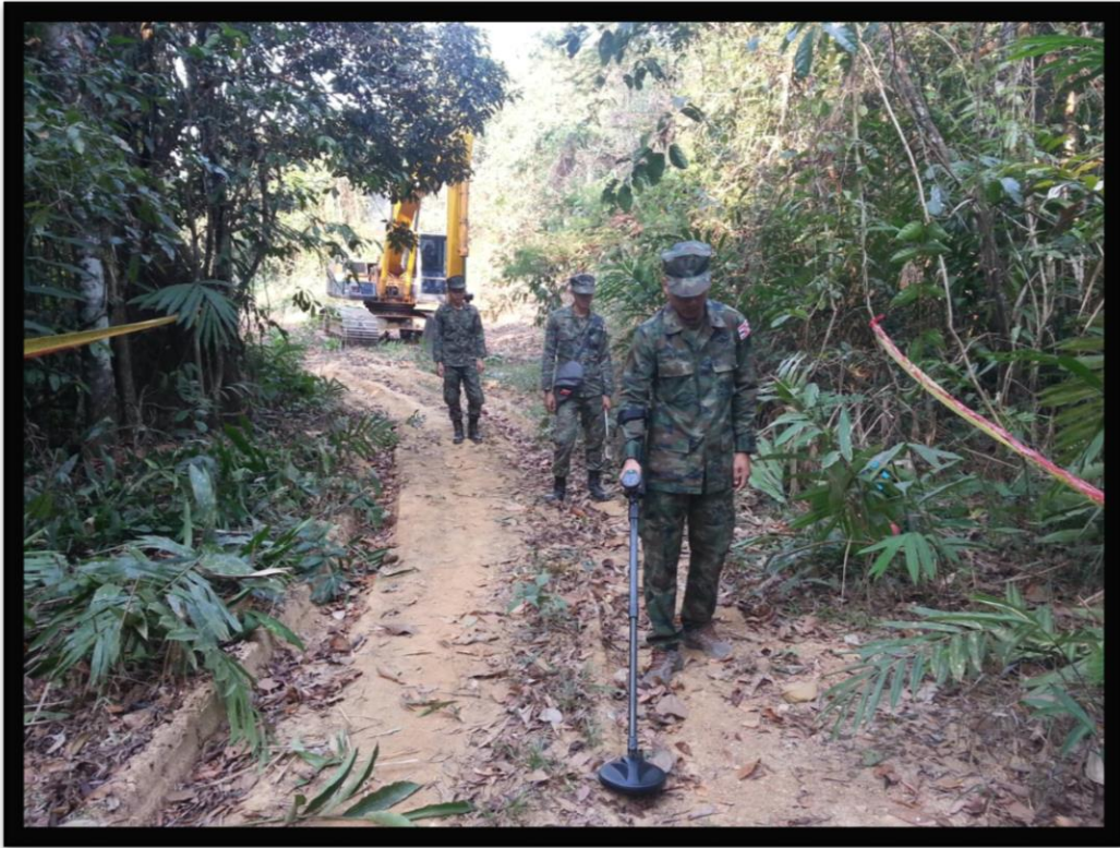
ขั้นตอนที่ 1 ใช้ชุดตรวจค้นตรวจค้นวัตถุระเบิดเปิดช่องทางที่ต้องการปรับปรุงให้ปลอดภัยจากทุ่นระเบิด
